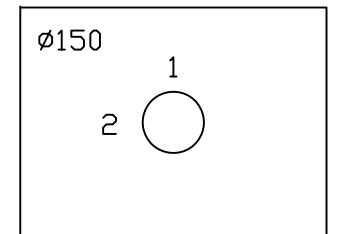
д - КАБЛОВСКА КАНАЛИЗАЦИЈА Ø150 У ЈЕДНОМ РЕДУ СА 2 ОТВОРА
