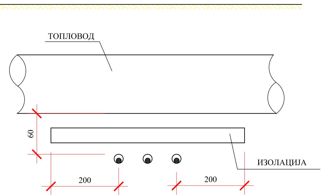
ПРЕСЕК 2 - 2
