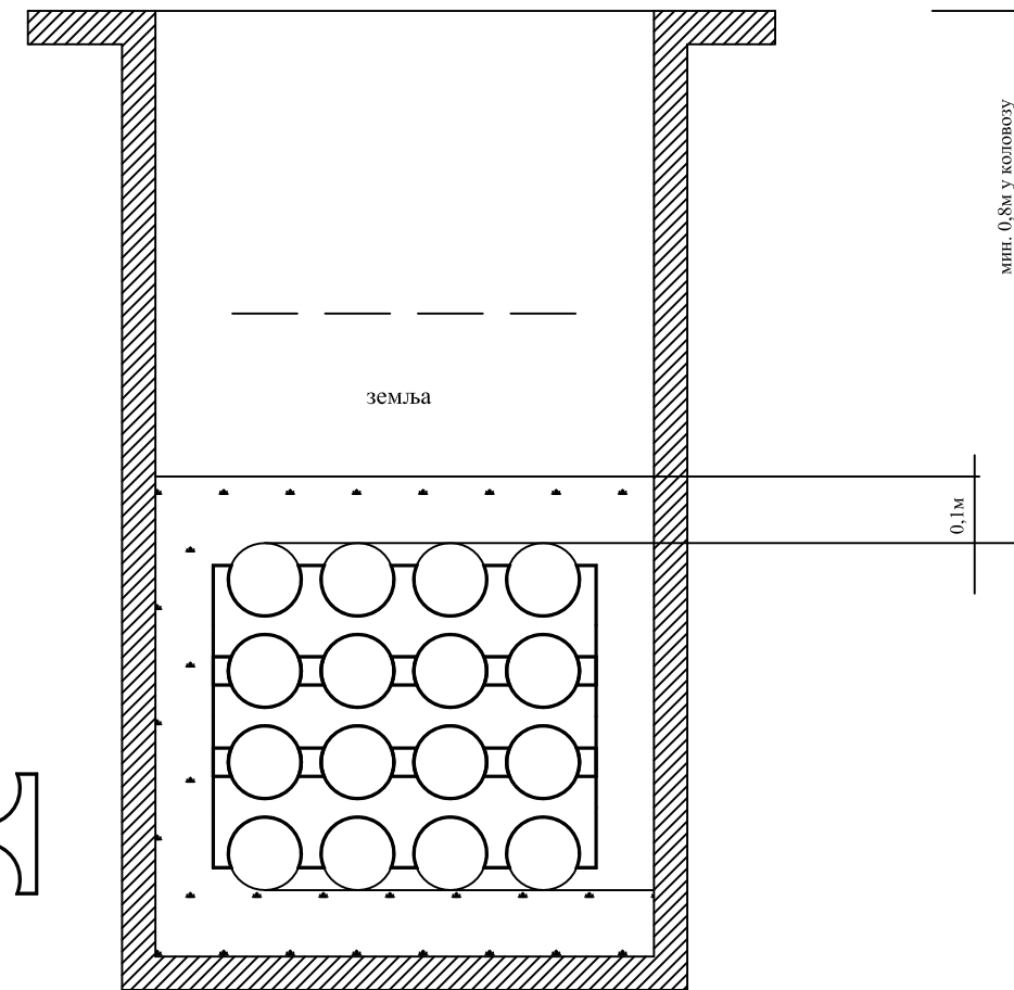
Канализација од ПВЦ цеви у коловозу
