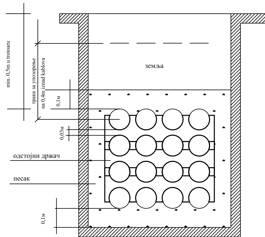
Канализација од ПВЦ цеви у тротоару
