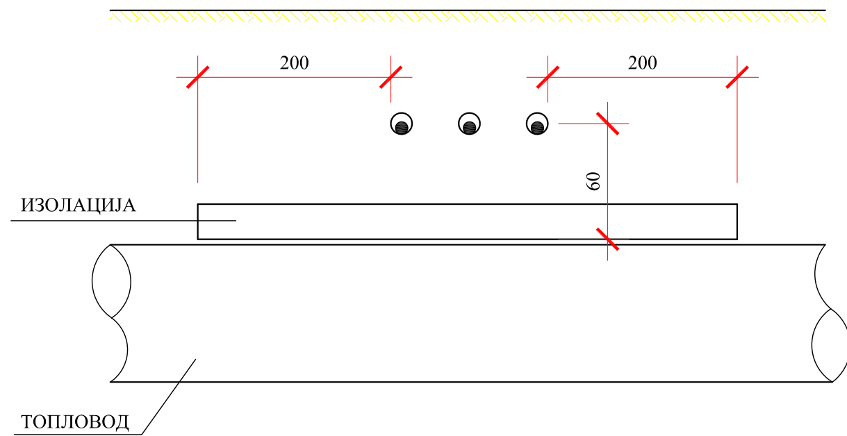
ПРЕСЕК 1 - 1
