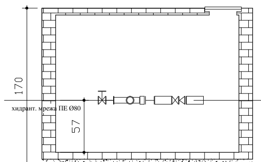
пресек А-А
