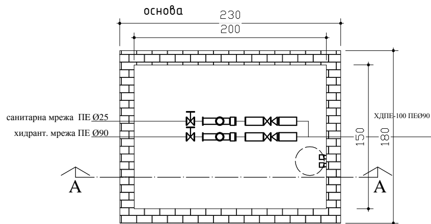
водомер Ø25-мокри чвор
