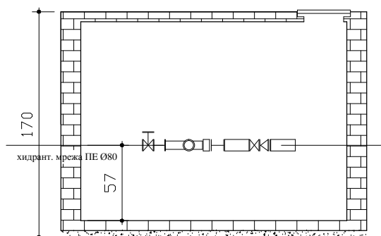
пресек А-А
