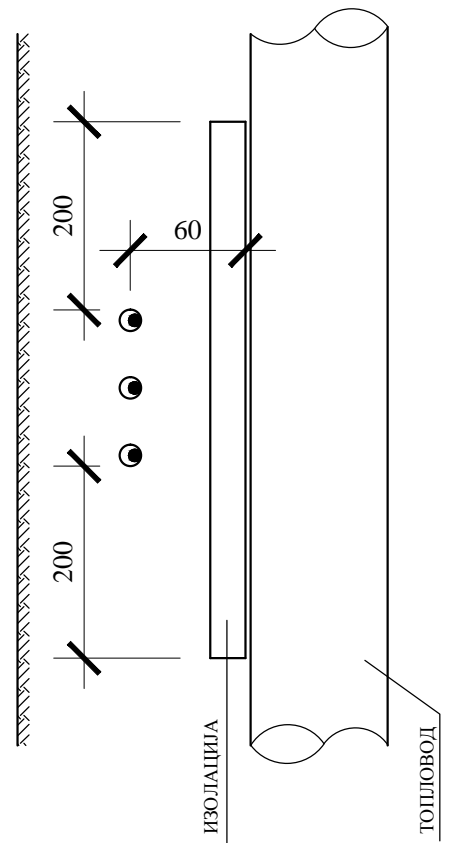
ПРЕСЕК 1 - 1
