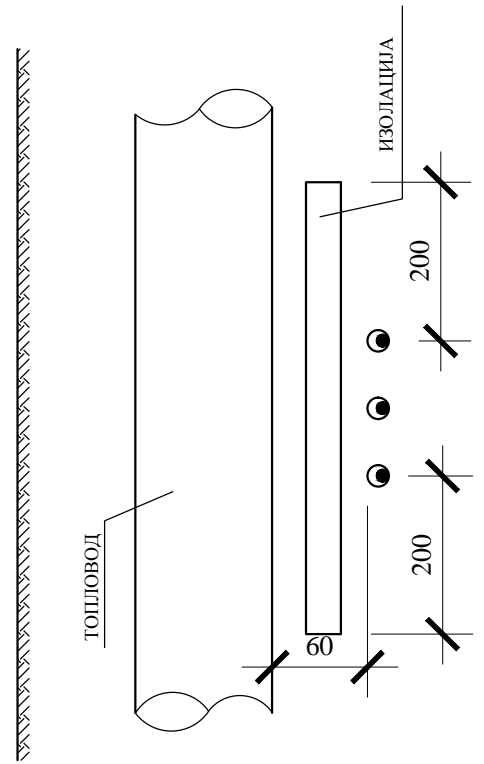
ПРЕСЕК 2 - 2
